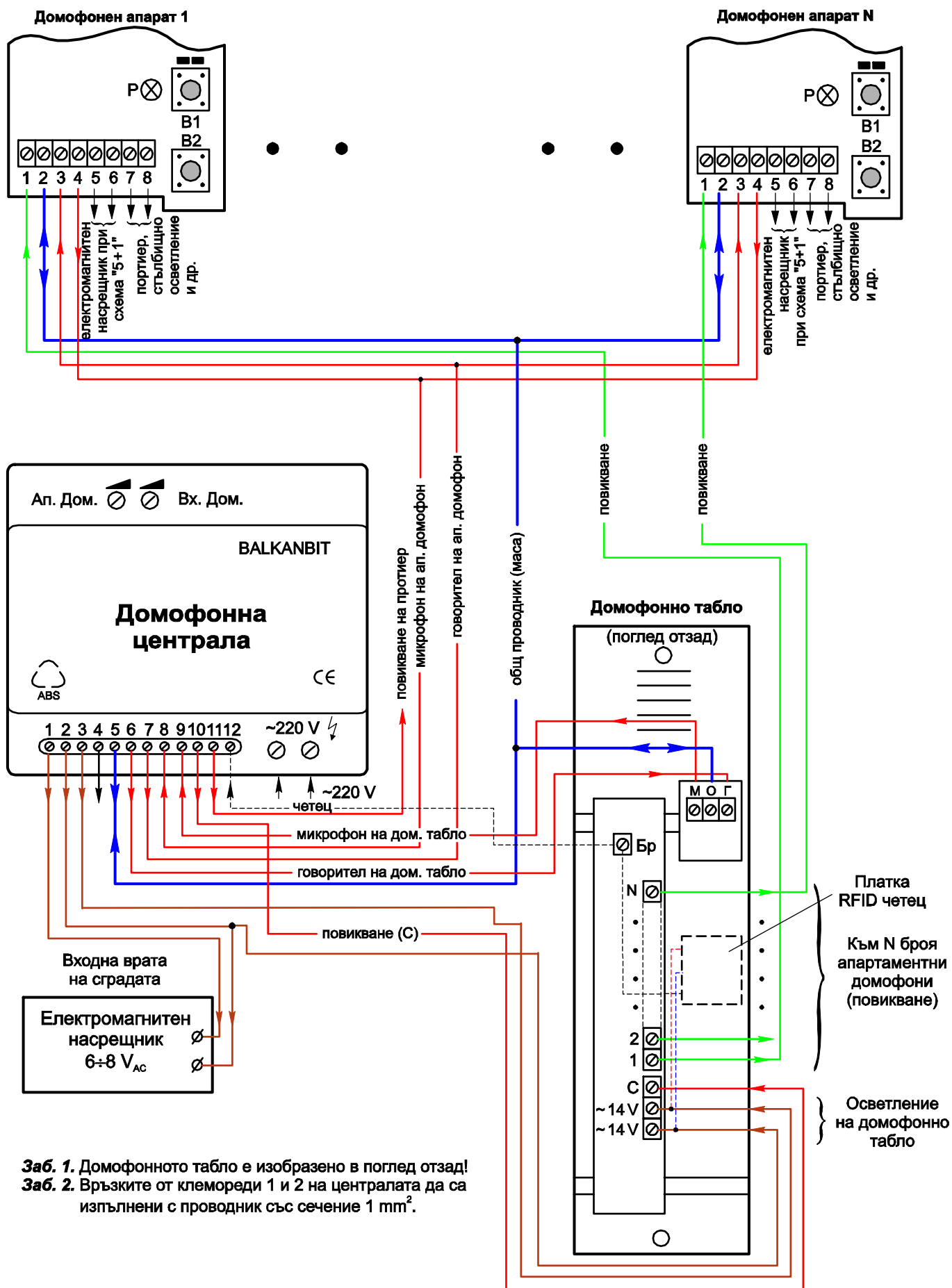
Схема на свързване (3 + 1)
